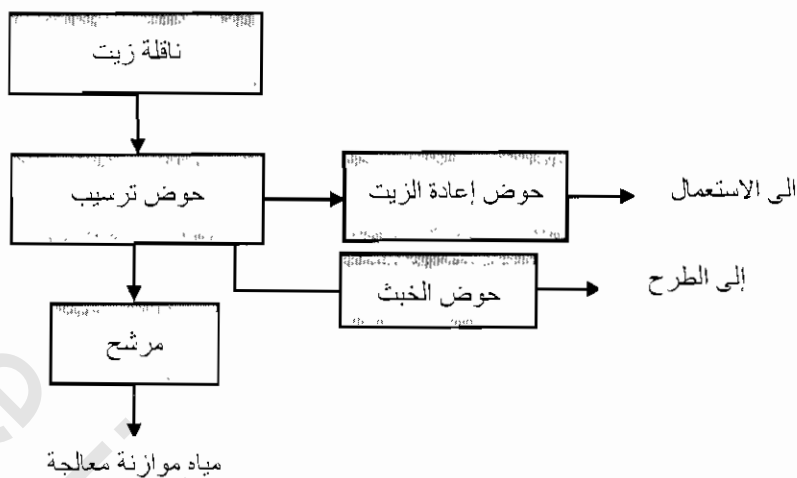
شكل (٧-١٣): مخطط لمعالجة مياه الاتزان للنقلات .
