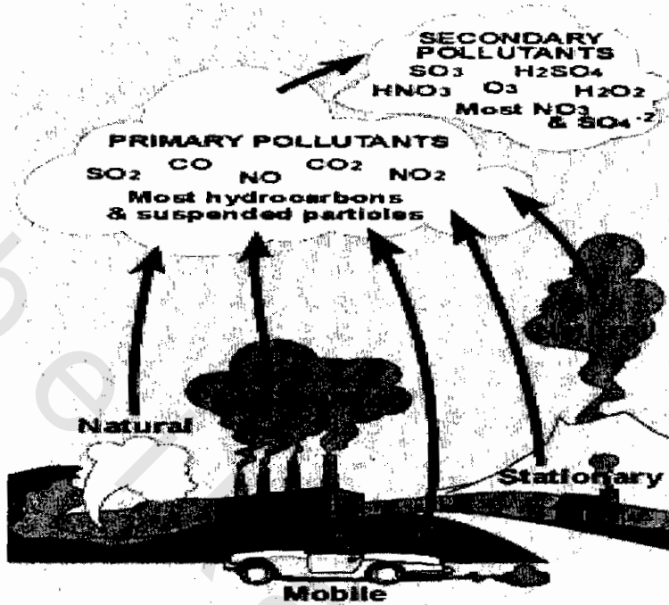
شكل (٢-١) الملوثات الأولية والثانوية للهواء
