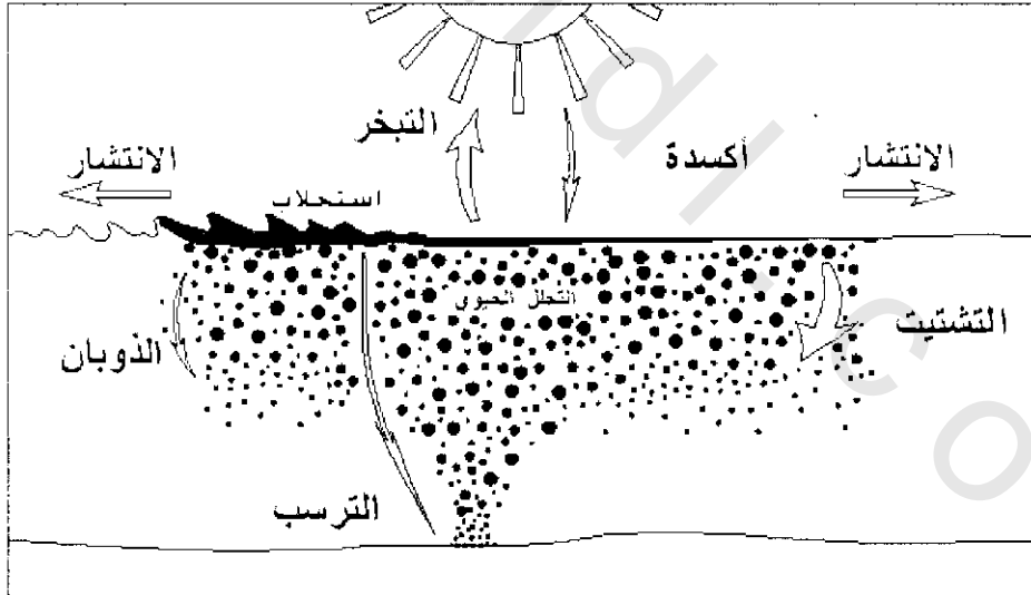
شكل (٤-٤): مخطط التلوث بزيوت البترول ومسار الزيت والركبات البترولية داخل وعلى سطح البحر.
