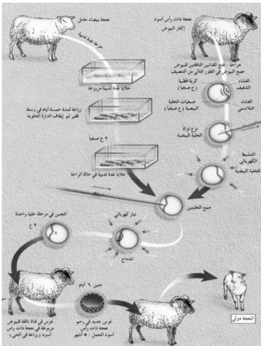
شكل رقم (١٢-١) يبين خطوات استساخ النمجة دوللي
