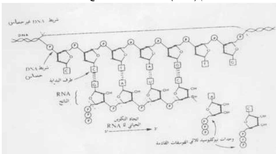
الشكل رقم (٢-١٤) يبين عملية استنساخ الشريط الحساس
