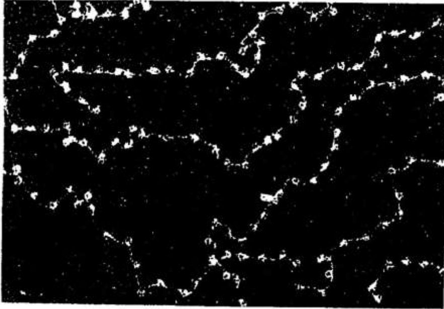
الشكل رقم (٣-٢) يبين صورة بالمجهر الالكتروني تظهر فيها النيوكليوسومات مأخوذة من مزرعة نسيجية للفأر ( عن حيدر والحاسي ، ٢٠٠٤ )
