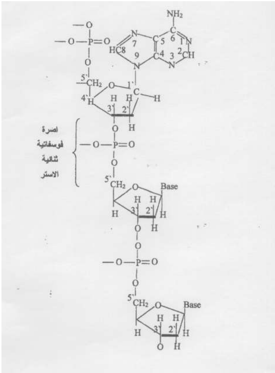
الشكل رقم (٢-٤) يبين الاواصر الفوسفاتية ثنائية الاسر التي تربط النيوكليوتيدات في شريط الـ DNA
