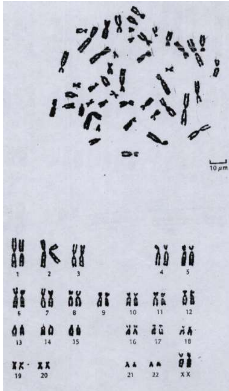
شكل رقم (٨-٥) يبين الهيئة الكروموسومية الطبيعية في الانسان
