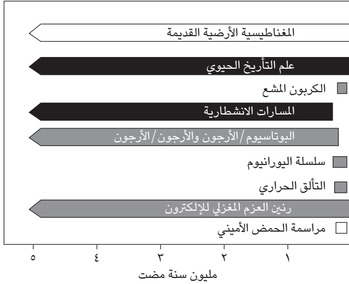
شكل ٢-٣: بعض الطرق المُستخدمة في تأريخ حفريات أشباه البشر والفترات الزمنية التي تغطيها.
