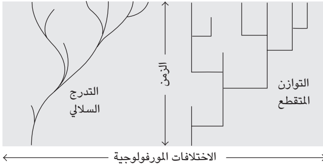
شكل ٤-١: الفرضيتان الأساسيتان «التردد السلالي» و«التوازن المتقطع» بشأن توقيت التغير المورفولوجي الذي يحدث في أثناء عملية التطوُّر.
