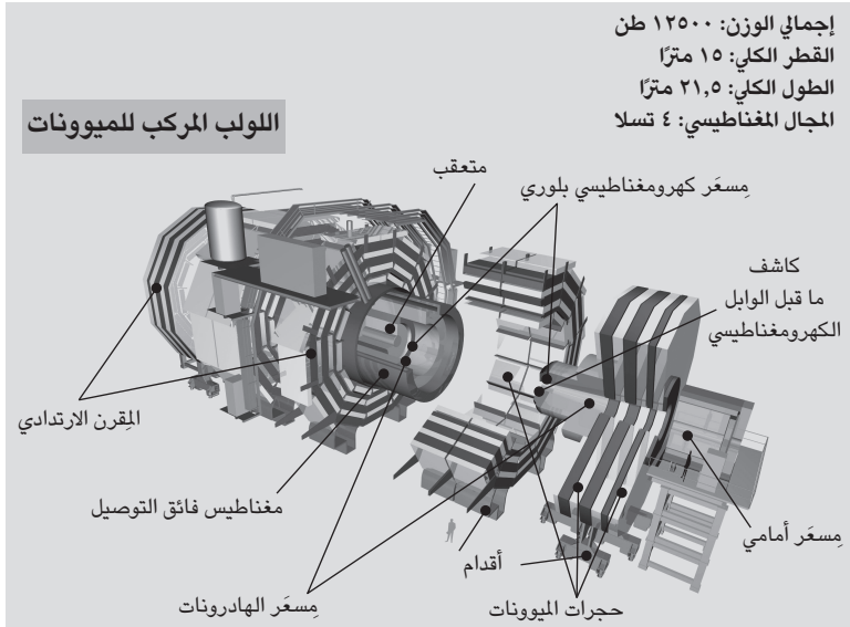
شكل ١٣-٥: صورة بالكمبيوتر للولب المركب للميونات مُفكَّكًا لعرض كلِّ مكوّن من مكونات الكاشف (الرسم مُقدّم من سيرن وتجربة اللولب المركب للميونات).
