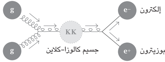
شكل ١٧-١٤: في نماذج راندل-ساندرم، يمكن أن ينتج جرافيتون كالوزا-كلاين ويتحلل داخل الكاشف إلى جسيمات مرئية، مثل الإلكترون والبوزيترون.
