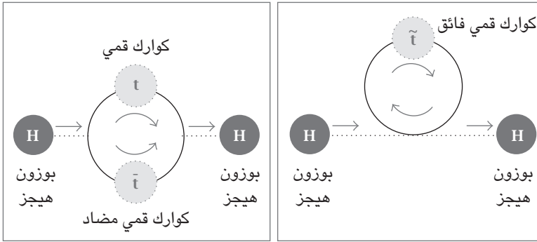
شكل ١٧-٣: في نموذج التناظر الفائق، إسهامات جسيمات التناظر الفائق الافتراضية تلغي إسهامات جسيمات النموذج القياسي في كتلة بوزون هيجز. على سبيل المثال، مجموع الإسهامات من الرسمين الموضحين أعلاه يساوي صفرًا.
