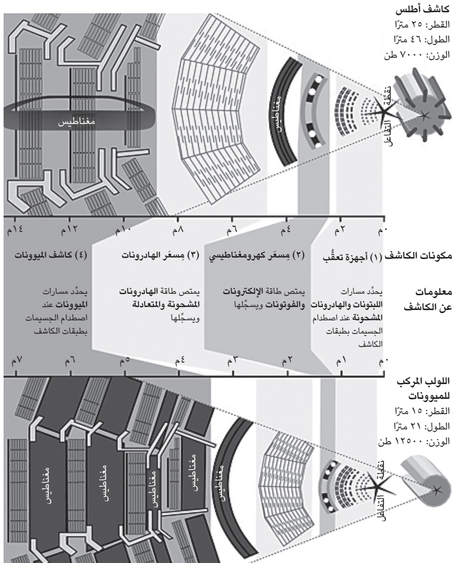
شكل ١٣-٤: مقاطع عرضية لكاشفي أطلس واللوب المركب للميوانات. يُرجى ملاحظة أن الأحجام الكلية بالرسم لا تعبر عن الأحجام الحقيقية.
