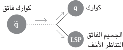
شكل ١٧-٤: يمكن للكوارك الفائقة أن يتحلل إلى كوارك والجسيم الفائقة التناظر الأخف.
