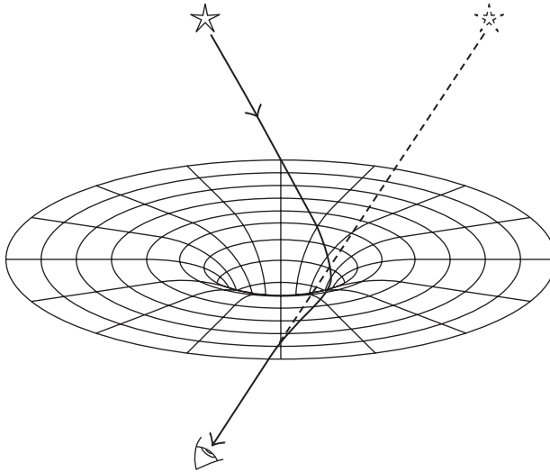
شكل ٢-٧: تمثيل للطريقة التي يمكن أن ينحني بها الضوء القادم من نجم بعيد بفعل انحناء الفضاء الذي تسببه الشمس.
