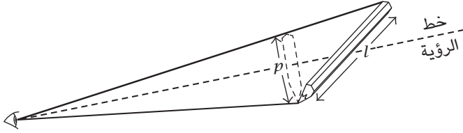
شكل ١-١: القلم الرصاص ذو الطول l له طول منعكس p متعامد على خط الرؤية للراصد.
