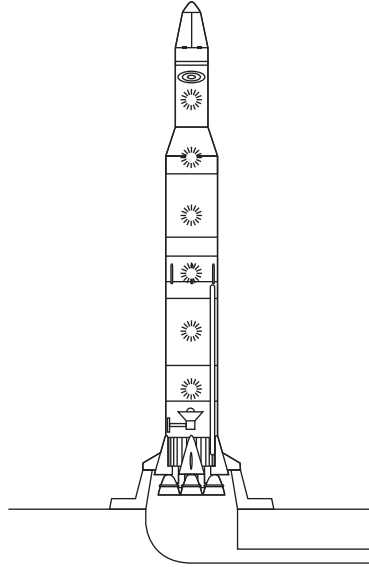
شكل ٢-٣: نبضات منتظمة من الضوء تُرسل من مؤخرة المركبة إلى مقدمتها، بينما تنتصب المركبة على نحو رأسي على منصة الإطلاق.
