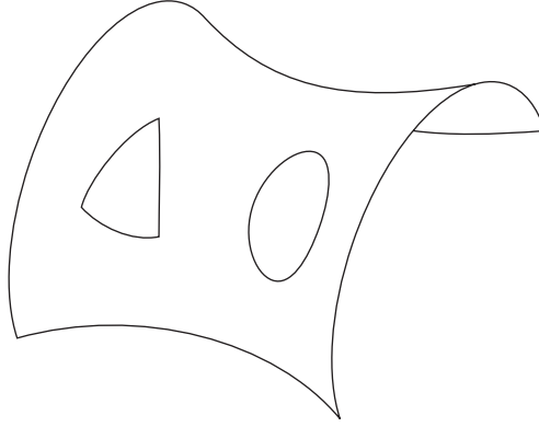
شكل ٢-٩: السرج شكل آخر تكون الهندسة داخل سطحه مختلفة عن الهندسة على سطح مستوي.
