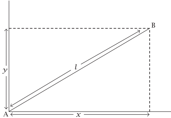
شكل ١-١٢: يمكن التعبير عن الطول l من خلال العنصرين x و y ، وذلك وفقًا لنظرية فيثاغورس.
