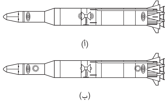
شكل ٦-١: من منظور رائد الفضاء، النبضتان المنطقتان في الآن عينه من منتصف المركبة تصلان إلى طرفي المركبة على نحو متزامن.
