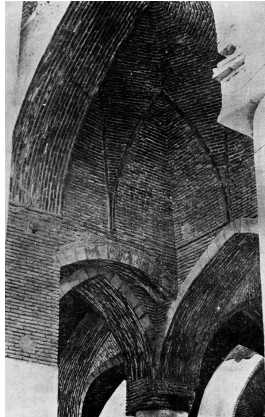
شكل ٤: قبو وعقود في المسجد الجامع بأصفهان (عن بوب).
