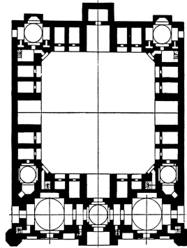
شكل ٢٦: تخطيط مدرسة خرجود (عن بوب).
