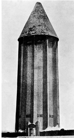
شكل ٦: جنبد قابوس في جرجان، مؤرخة ٣٩٧هـ/١٠٠٦م (عن بوب).
