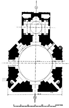
شكل ٢٥: تخطيط ضريح الجايـتو في مدينة سلطانية (عن جودار).
