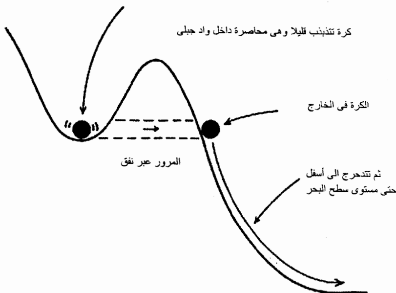
شكل رقم (٢٤) السلوك النفقى على المستوى الكمي
