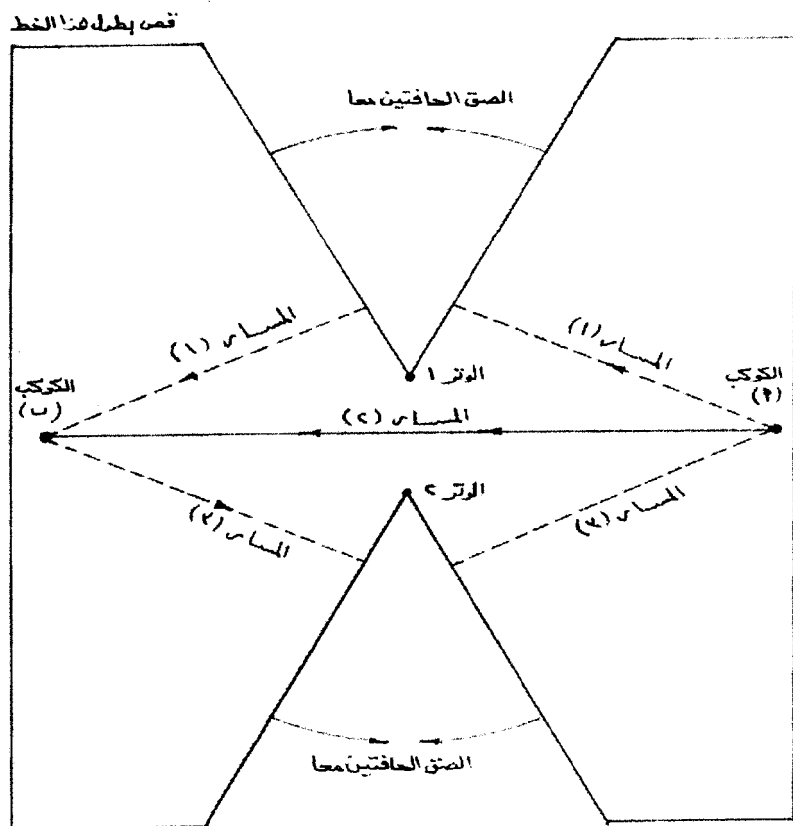
شكل رقم (١١) الفضاء حول وترين كونيين
