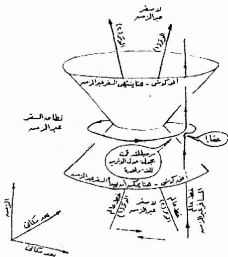
شكل رقم (١٤) نطاق السفر عبر الزمن حول وترين كونييين
