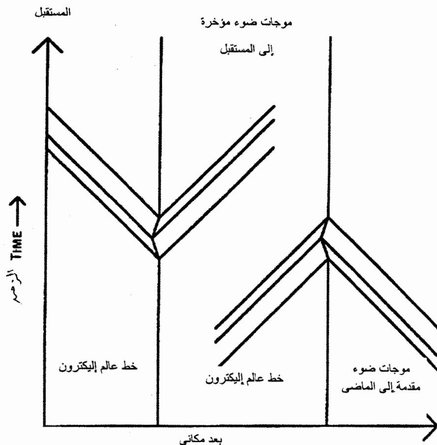
شكل رقم (٢٨) سهم الزمن.
