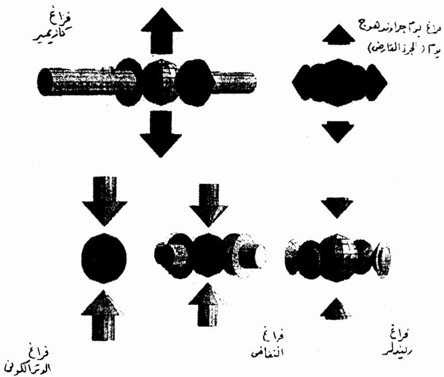
شكل رقم (١٧) أنواع الفراغات
