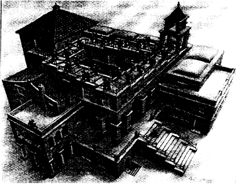
شكل رقم (١٣) الصعود والهبوط (١٩٦٠) للرسم م.ك. إشر
