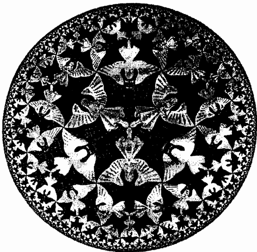
شكل رقم (٢٣) : حد الدائرة (١٩٦٠) للرسم م.ك. إشر يوضح الشكل كونا مفتوحا سالب الانحناء.
