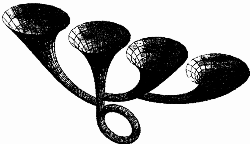
شكل رقم (٢٧) الكون خالف نفسه
