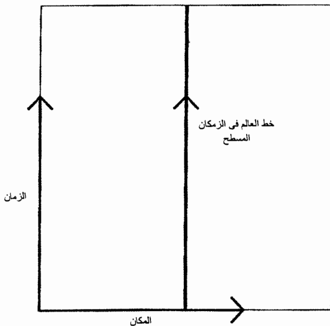
خط العالم في الزمكان المنحني
