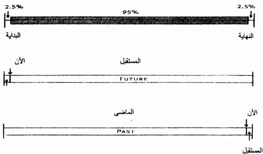
شكل (٣١) برهنة مبدأ كوبرنيكوس (باحتمال ٩٥٪)
