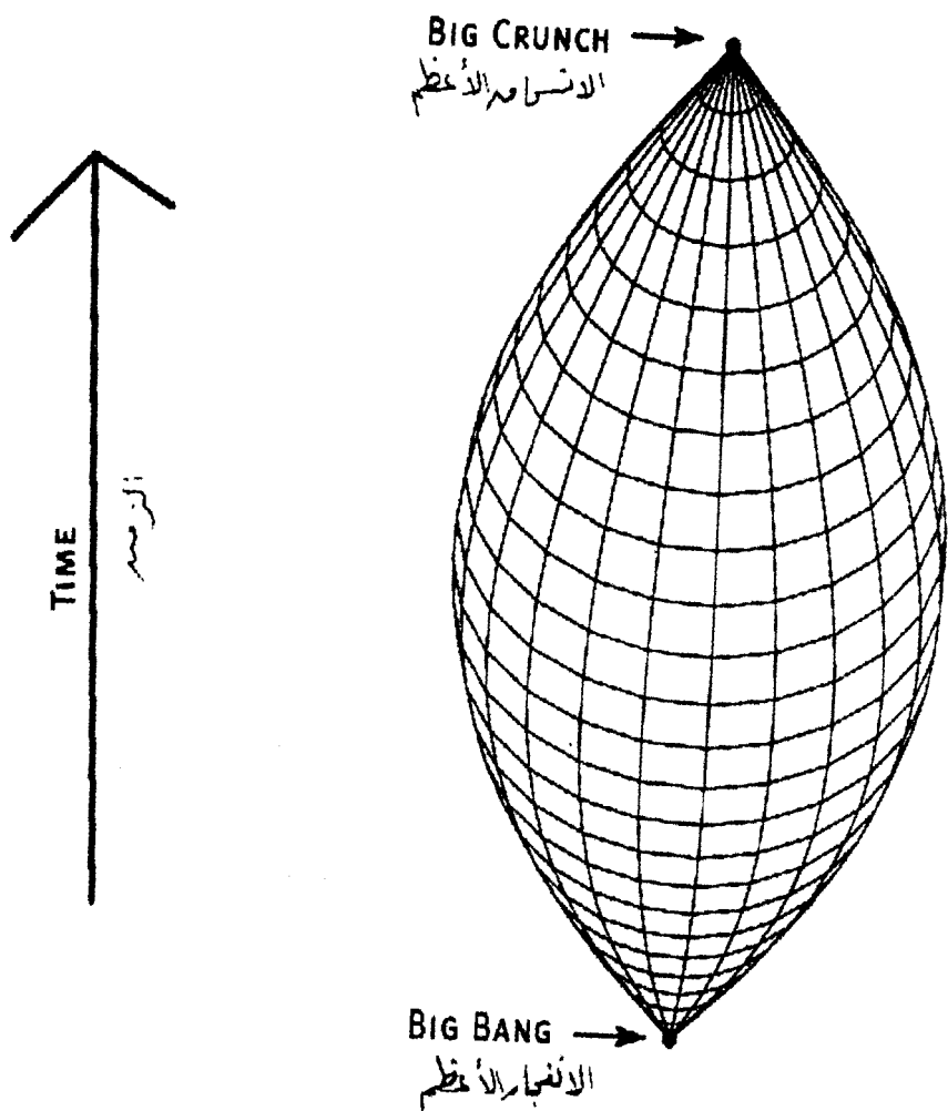
شكل رقم (١٩) نموذج فريدمان للكون المغلق ثلاثي الكرات
