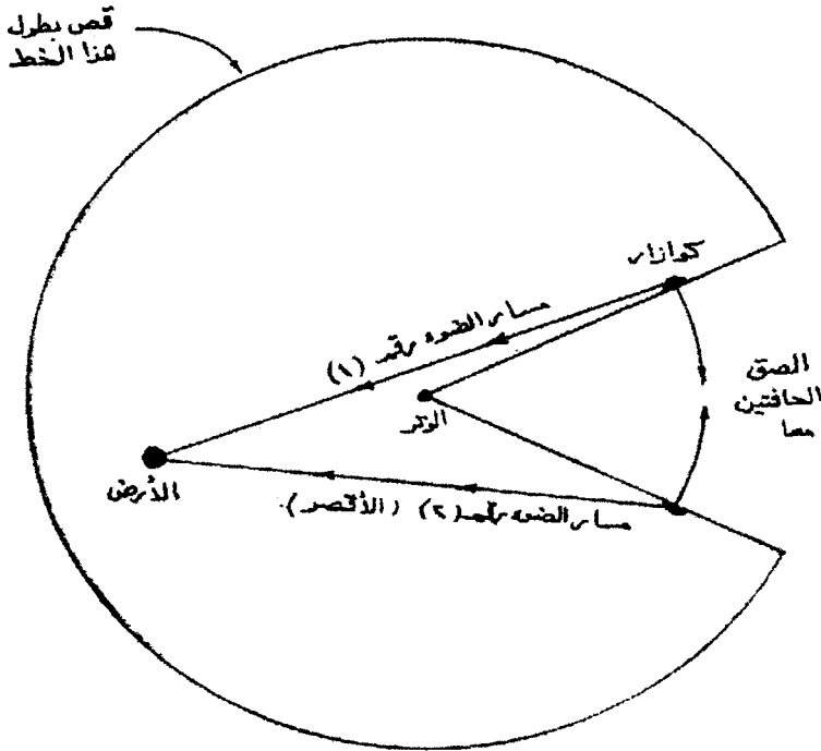
شكل رقم (١٠) الفضاء حول وتر كوني
