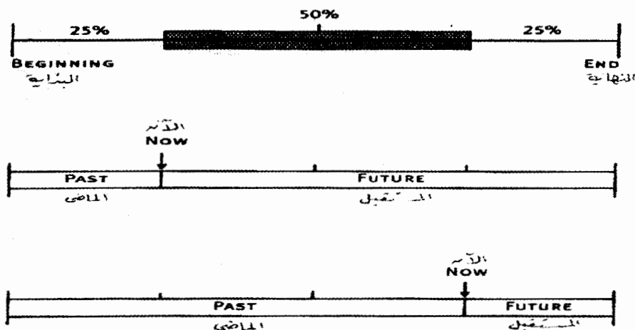
شكل رقم (٣٠) المسألة الكوبرتيكية احتمالية ٥٠٪
