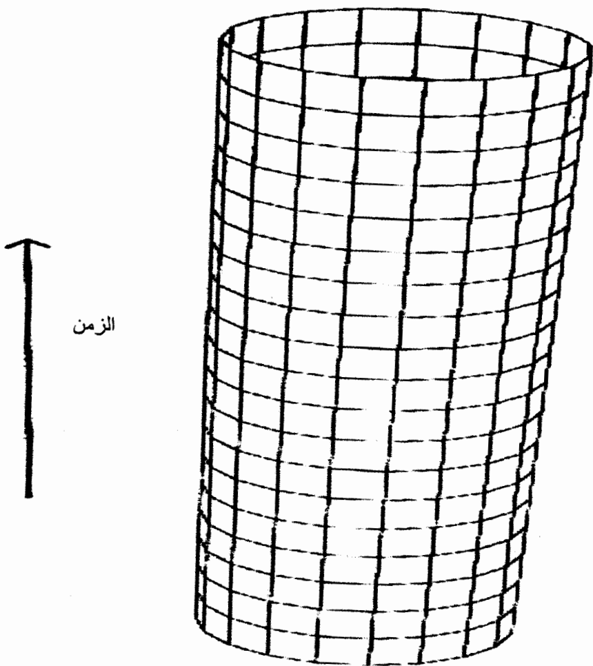
شكل رقم (١٨) كون أينشتاين الاستاتيكي
