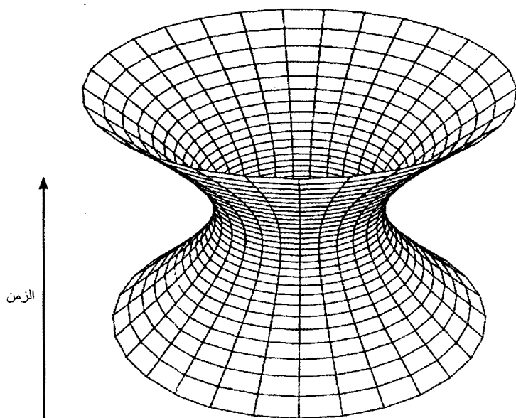
شكل رقم (٢١) - زمكان دى سىتر
