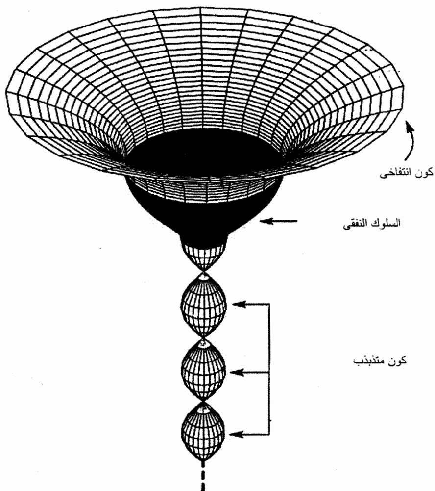
شكل رقم (٢٦) يؤول الكون المتذبذب الصغير في النهاية إلى السلوك النفقي.
