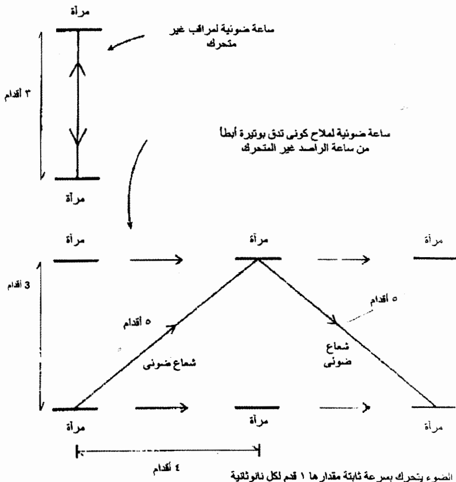
شكل رقم (3): اختلاف الساعات الضوئية
