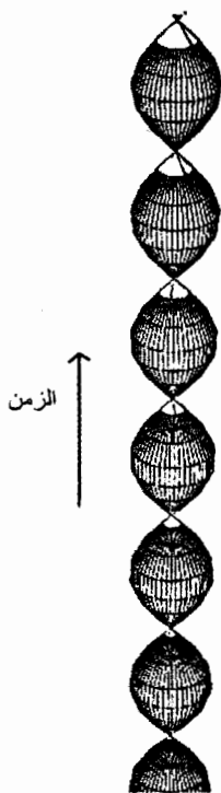
شكل رقم (٢٠) الكون المتذبذب
