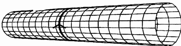
يتقوس الزمكان في شكل أسطوانة مكونة منحنى مغلقا (زماني المسمة)
